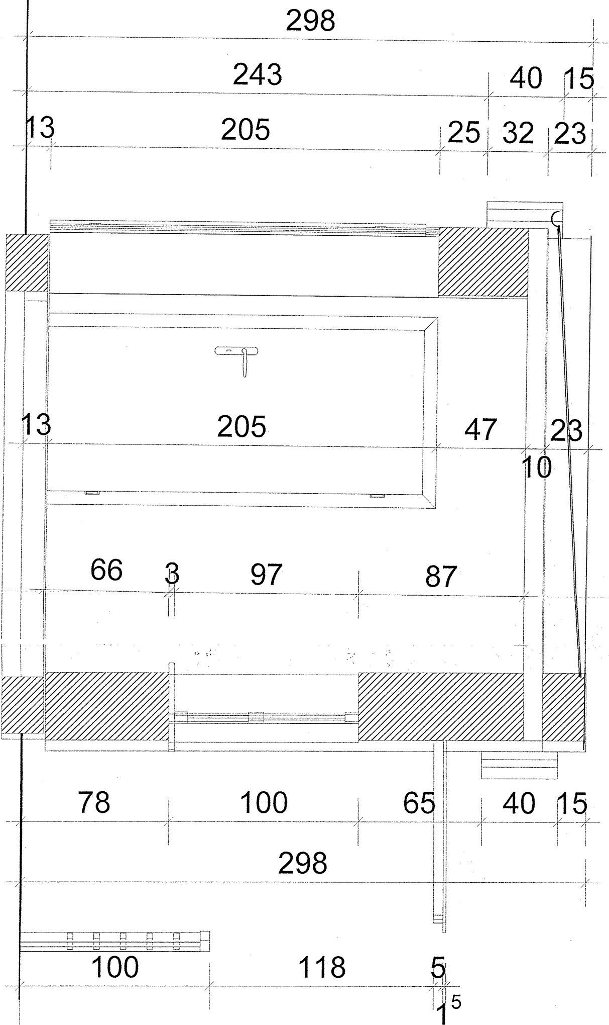
PRZEKRÓJ A : A OBIEKT KASOWY
